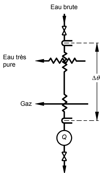
Figure 4 – Refroidisseurs connectés en série, deux fluides de refroidissements
